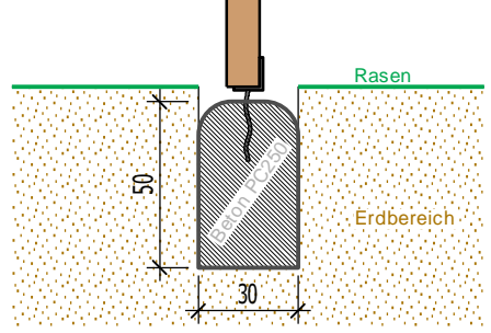
Detail: Fundament P-2
