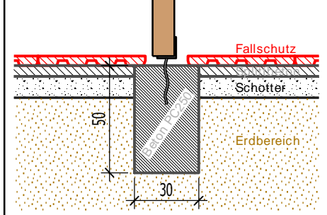
Detail: Fundament P-1
